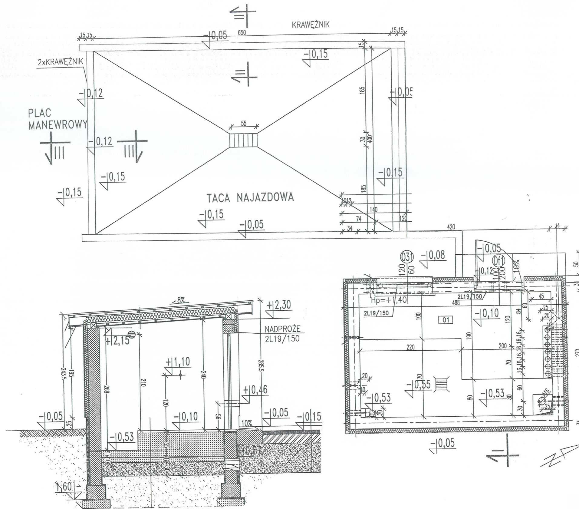
PRZEKRÓJ II 1:50
